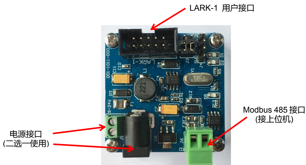
图 1. Modbus 转换板
